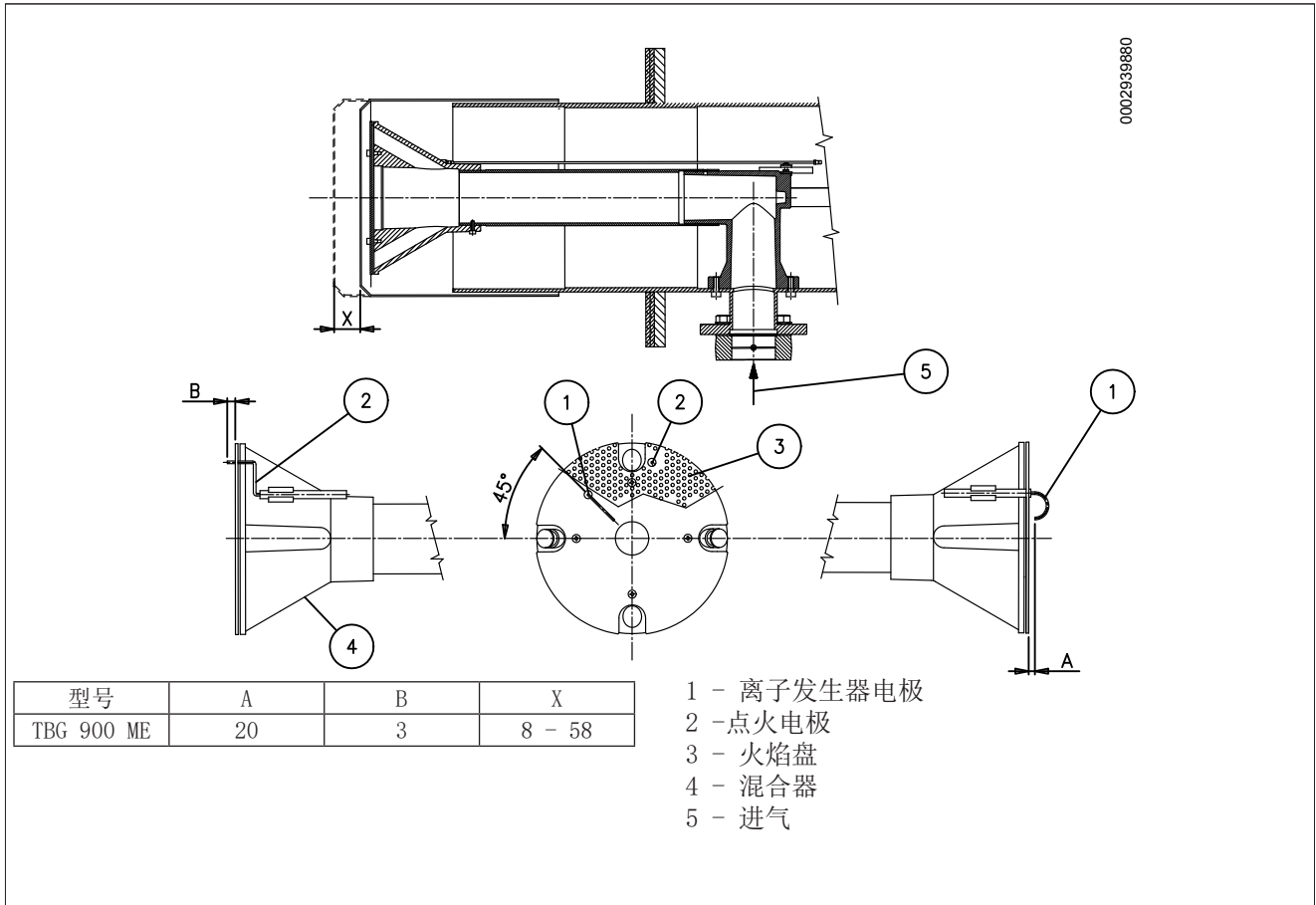
燃烧头-电机间距与燃烧头调节图
