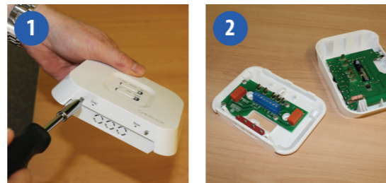
1 Ослабьте винты в нижней части приемника.
