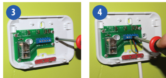
3 Прикрутите заднюю панель приемника к стене с помощью фитингов, поставляемых в комплекте.
